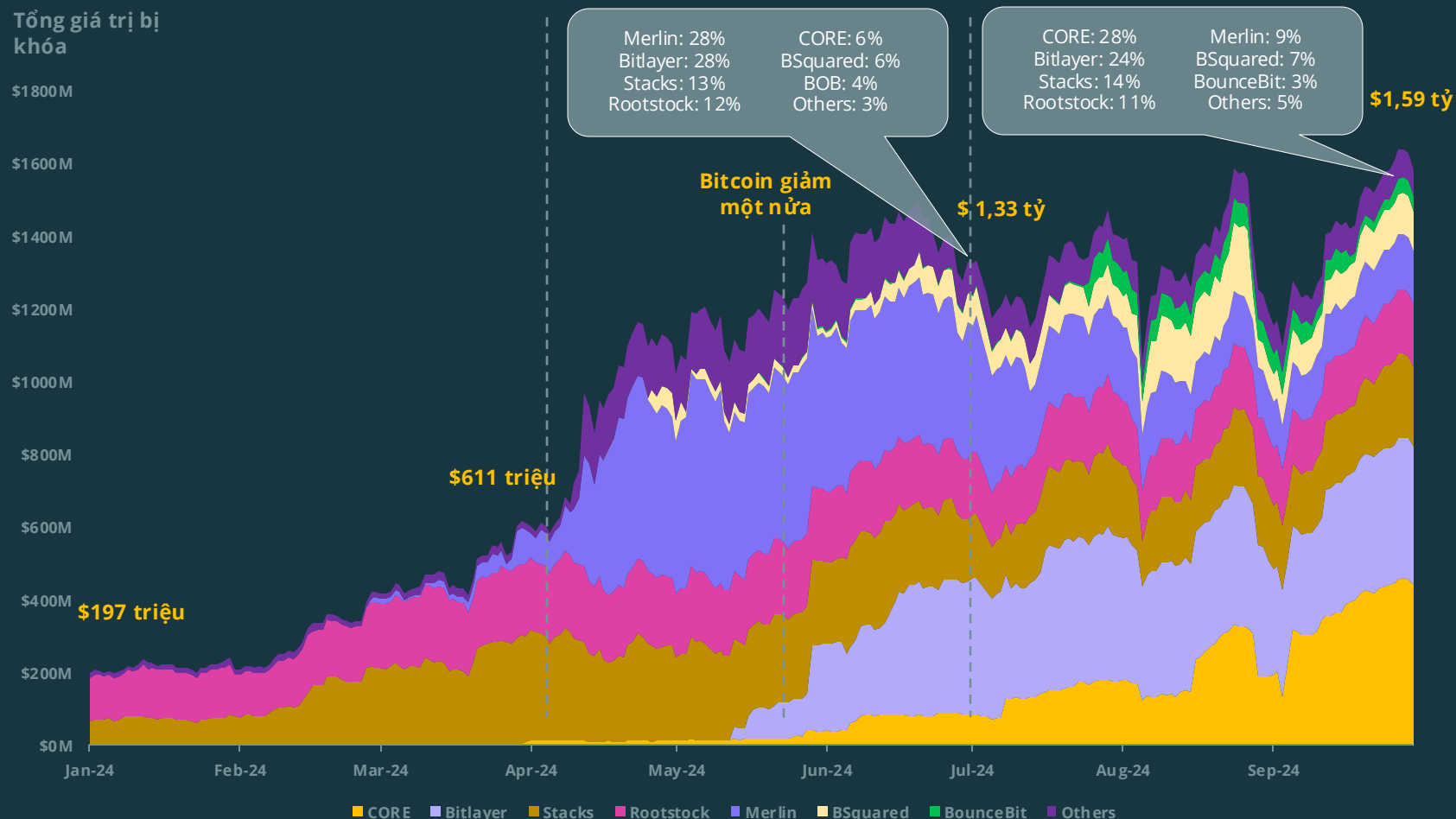
TVL trên Bitcoin Layer 2s (Quý 1 năm 2024 – Quý 3 năm 2024)
