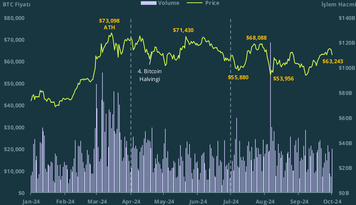
Bitcoin Fiyatı ve Spot İşlem Hacmi (2024 Q1 – 2024 Q3)
